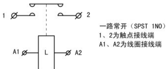
线路原理图
