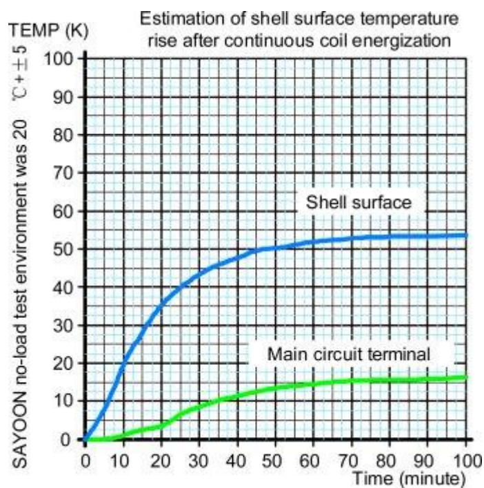
线圈温升曲线图
